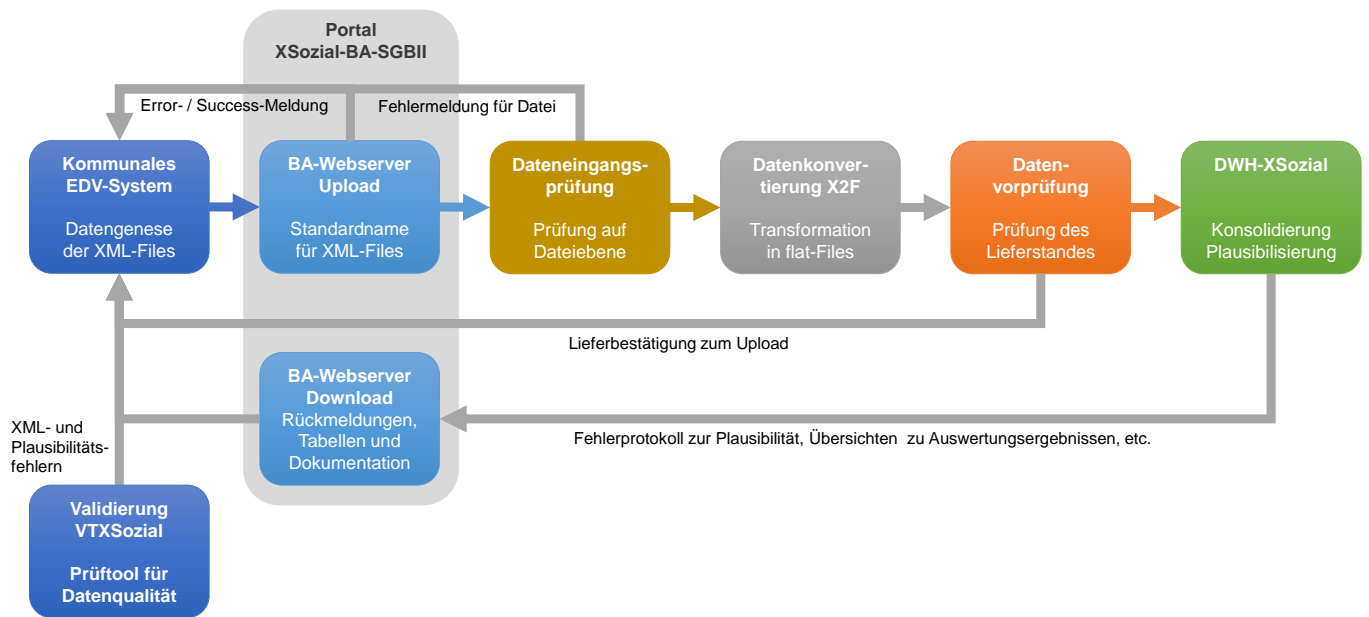
Abbildung 2 Übermittlungsprozess XSozial-BA-SGB II
