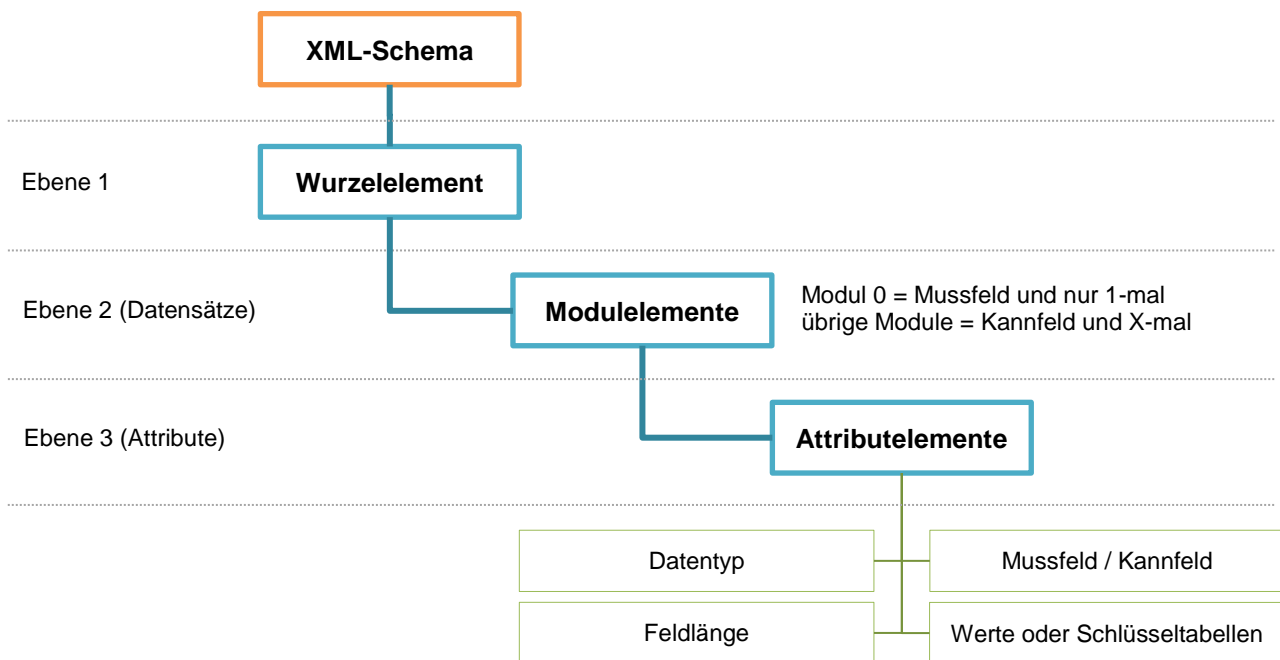
Abbildung 1 Aufbau und Struktur der XML-Datei (Baumstruktur)
